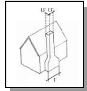
Chimney dimensions
